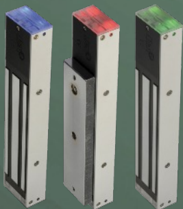
Ventouse 300 Kg 12/24V lumineuse V3SR ▶ 250 €
