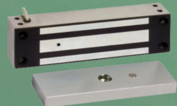
Ventouse 750 kg 12/24V. AVEC signal. EXT750-CTC ▶ 320 €
