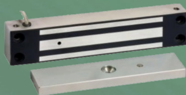
Ventouse 400 kg 12/24V. AVEC signal. EXT400-CTC ▶ 295 €
