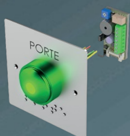
BP « Champignon » Buzzer+LED PB22MBBL ▶ 95 €
